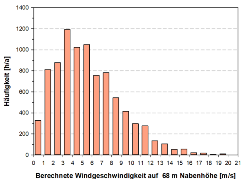
Abb. 3-18 – Häufigkeitsverteilung der berechneten Windgeschwindigkeiten am Referenzstandort auf Nabenhöhe des Rotors von 68 m (Datenquelle Windgeschwindigkeiten: Meteonorm, 2015)
