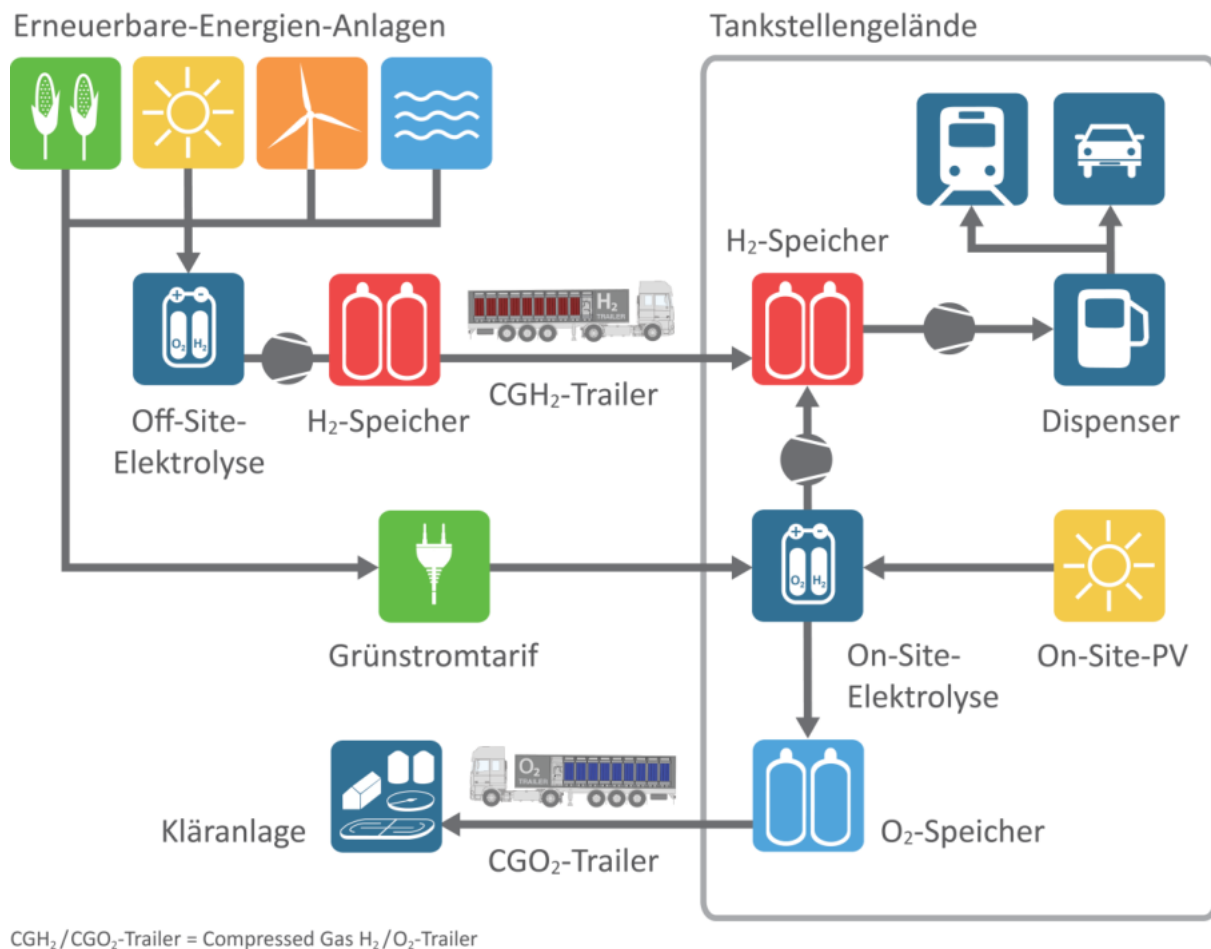
Abb. 2-1 – Mögliche Prozessketten zur H 2 -Bereitstellung für die Betankung von H 2 BZ-Triebwagen.
