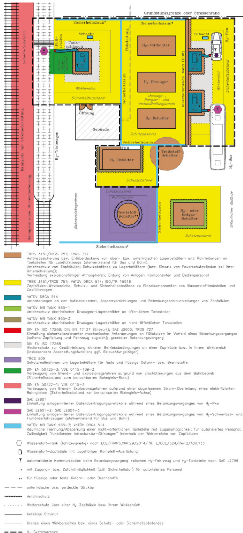
Abb. 2-6 – Geltungsbereiche relevanter technischer Regelwerke für Wasserstofftankstellen.
