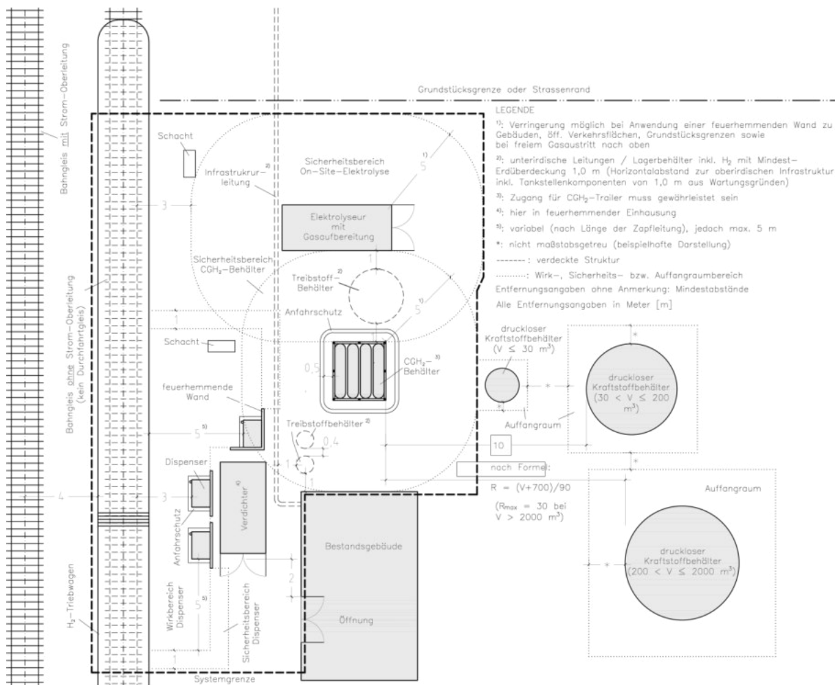
Abb. 2-7 – Prinzipskizze zu den einzuhaltenden Sicherheitsabständen einer Wasserstofftankstelle mit Onsite-Elektrolyse im Eisenbahnbetrieb entsprechend den analysierten technischen Regelwerken.
