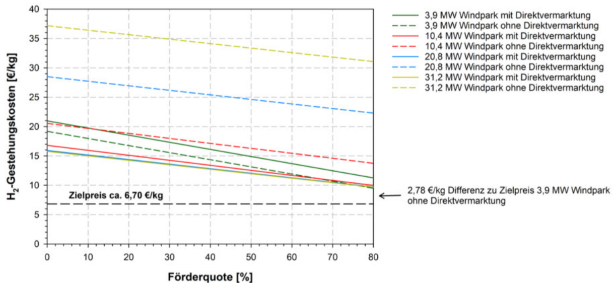
Abb. 4-3 - Wasserstoffgestehungskosten an der Tankstelle in Abhängigkeit von der Förderquote auf Investitionen, dem Vermarktungsmodell und der Windparkgröße bei einer Logistik mit Diesel-Zugmaschine.
