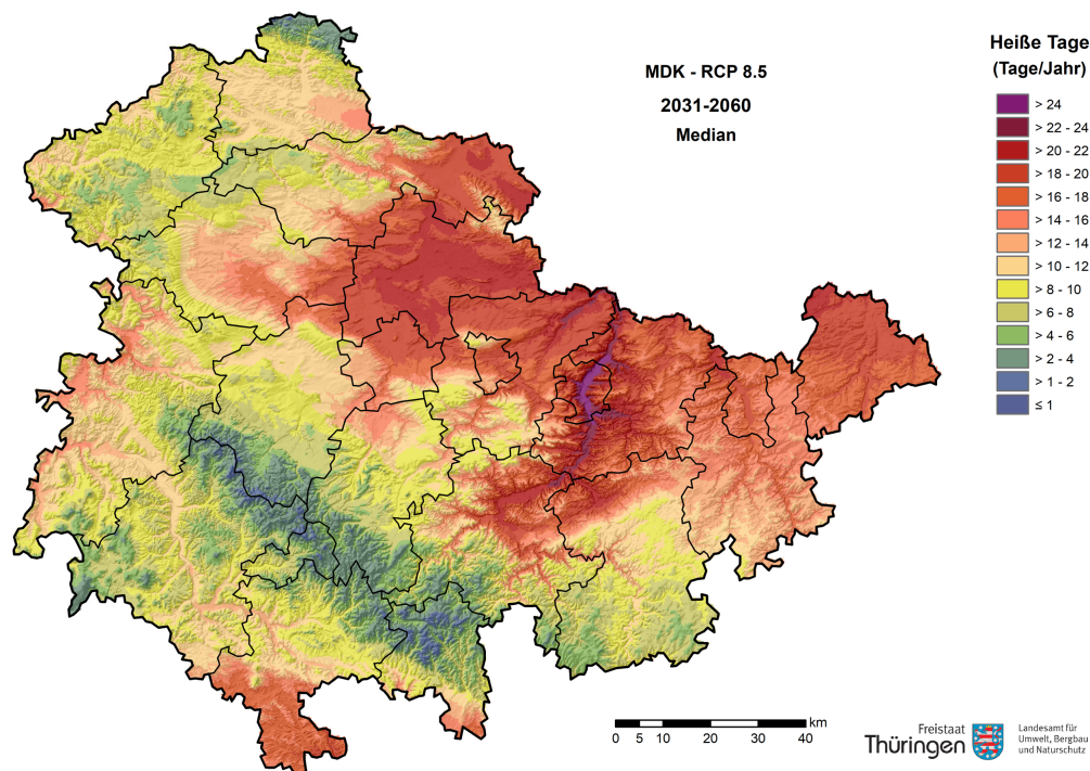
Abbildung 3: Zukünftige Entwicklung der jährlichen Anzahl der Heißen Tage in Thüringen in der Periode 2031–2060. Quelle: Kompetenzzentrum Klima am TLUBN
