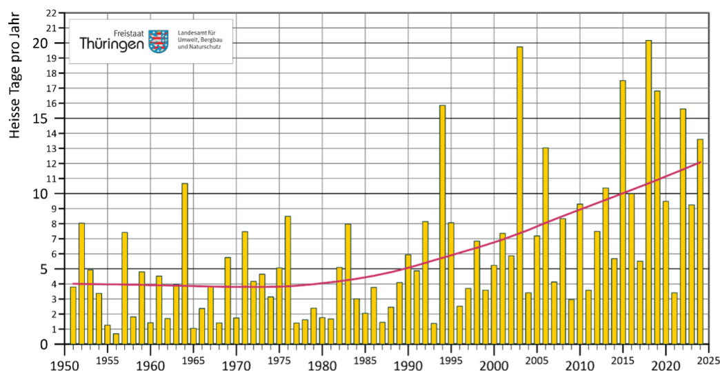
Abbildung 4: Beobachtete Entwicklung der jährlichen Anzahl der Heißen Tage im Flächenmittel Thüringens mit Darstellung einer Loess-Trendlinie (rot) (TLUBN 2025)
