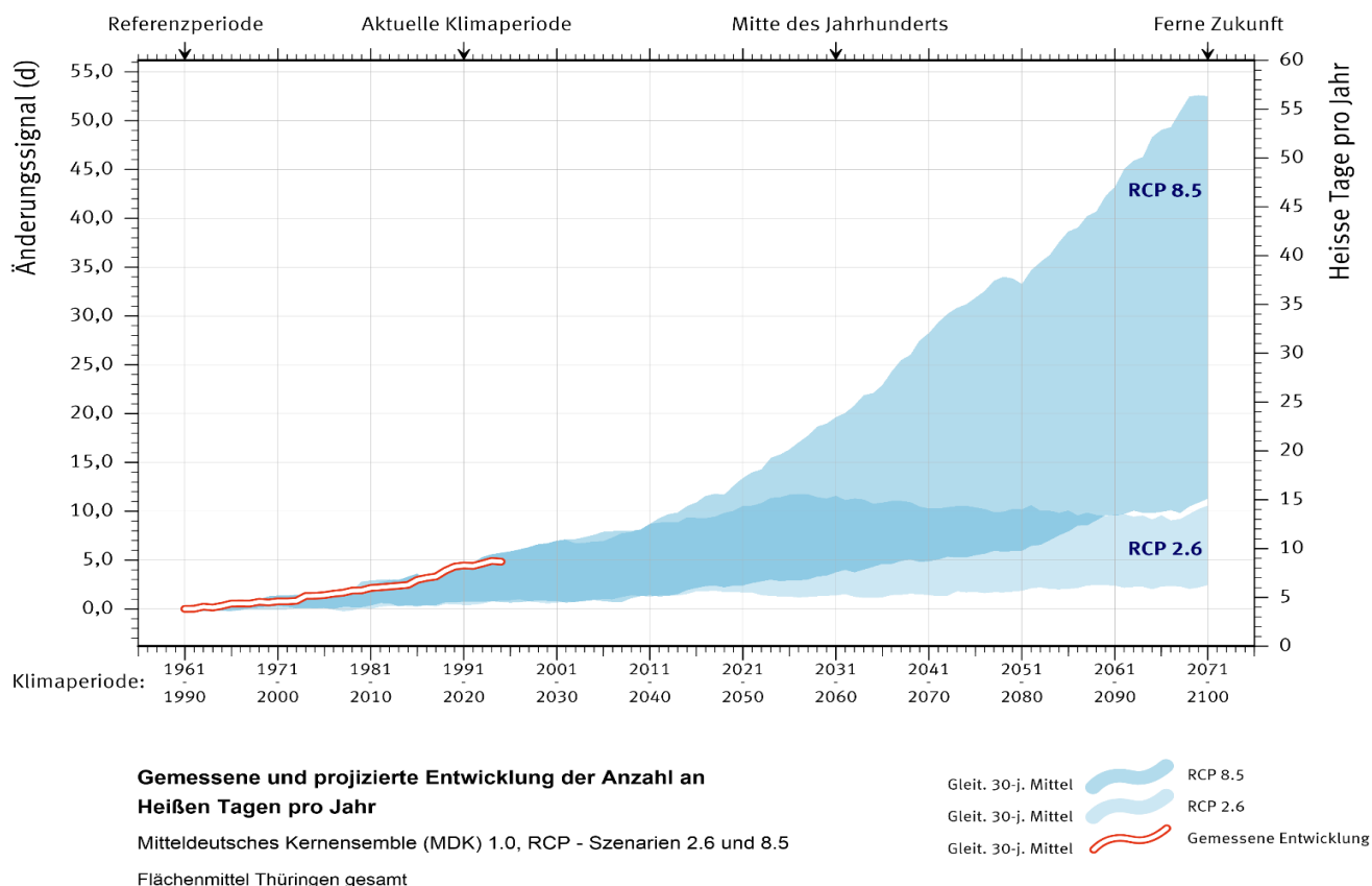
Abbildung 5: 30-jährige gleitende Mittel der aktuellen und zukünftigen Entwicklung der Anzahl Heier Tage pro Jahr in Thringen nach MDK 1.0 (Struve et al. 2020). Quelle: Kompetenzzentrum Klima am TLUBN
