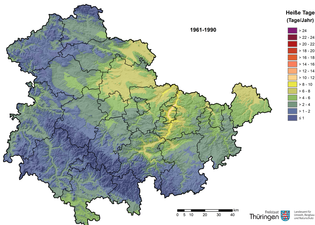
Abbildung 2: Mittlere jährliche Anzahl an Heißen Tage in Thüringen in der Referenzperiode 1961-1990 und der aktuellen Klimaperiode 1991-2020. Quelle:Kompetenzzentrum Klima am TLUBN
